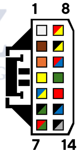
Rückansicht VL Digital Tyco/Hirschmann 14-poliger MQS- Stecker
